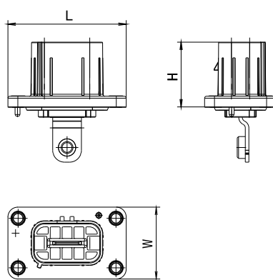
Tab Header
