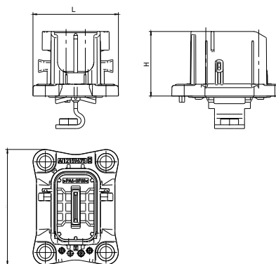
Tab Header
